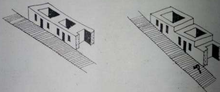
Fig 2.7 Maisons à patio en bandes (Amérique latine). A gauche : site plat. A droite : site en pente.
