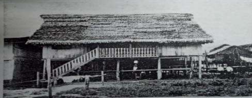
Fig. 2.2. Maison à Iquitos, Pérou (aire d'origine : Belén). Remarquer l'existence de solides murs pour préserver l'intimité, changement principal apporté par rapport à la maison de la fig. 2.1.
